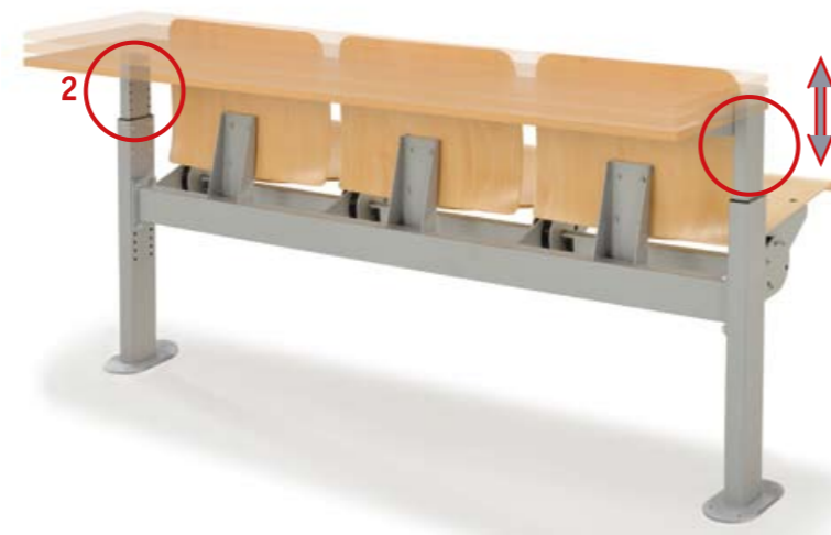
■ Ανεξάρτητη ρύθμιση ύψους επιφάνειας εργασίας. Independent working surface height adjustment.
