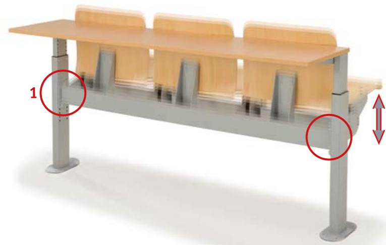
■ Ανεξάρτητη ρύθμιση ύψους καθίσματος Independent seat height adjustment.
